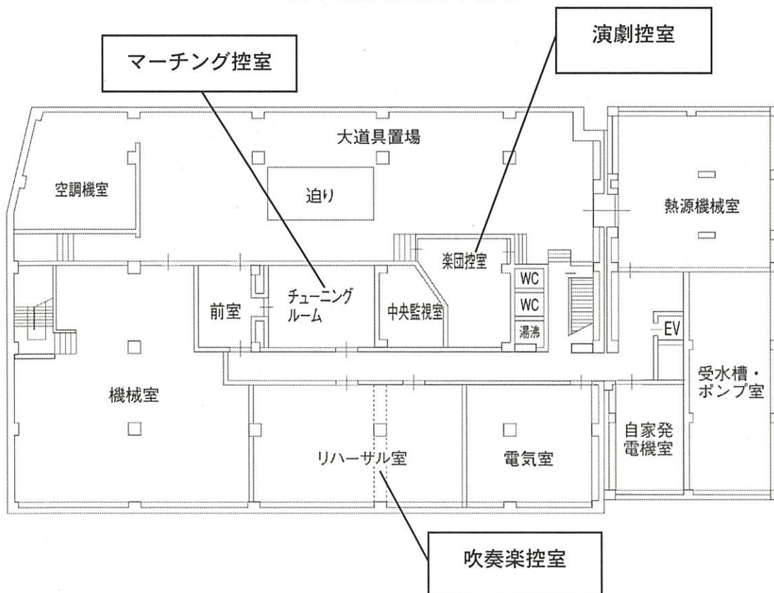
下関市民会館 地階平面図
