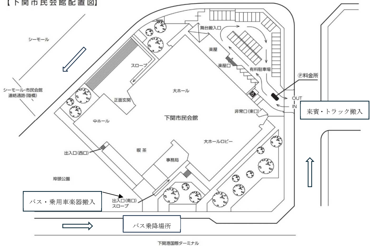
【下関市民会館配置図】
